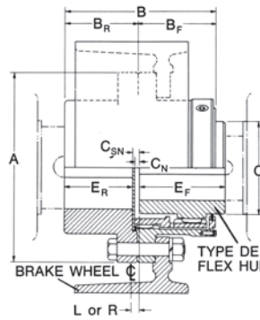
Type DEW
