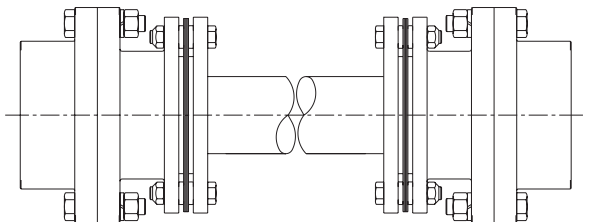
KD42
