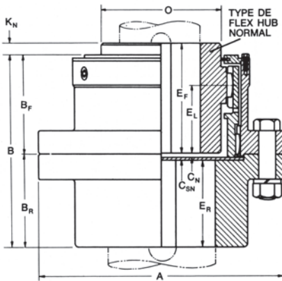
Type VDE
