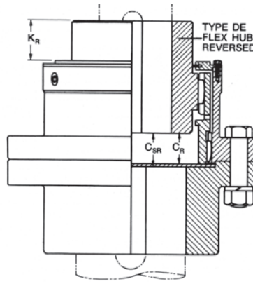
Type VDE
