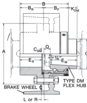
Type DMW
